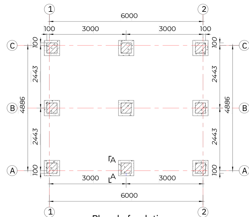
Plan de fondation
