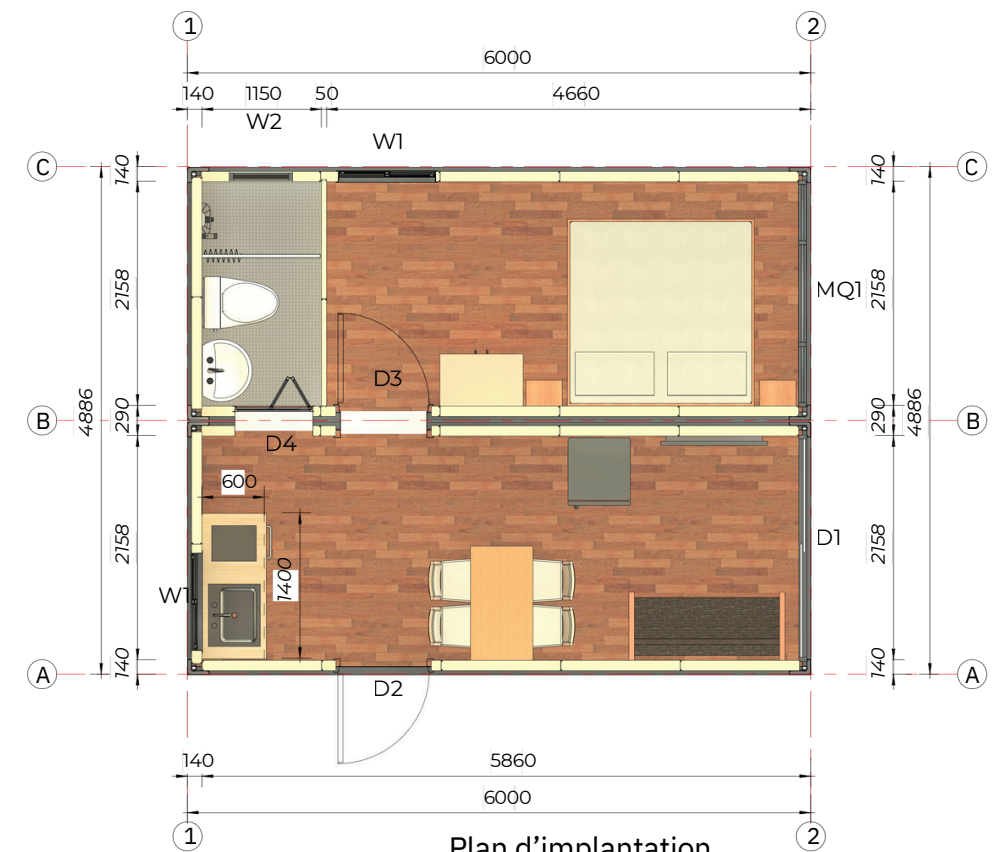
Plan d'implantation
