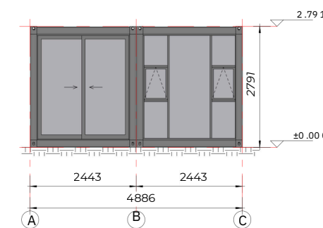
Élévation de la grille 2
