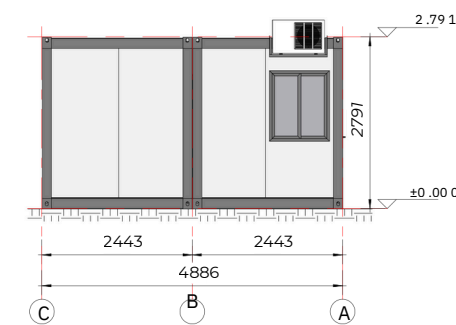
Élévation de la grille 1
