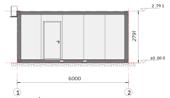
Élévation de la grille A
