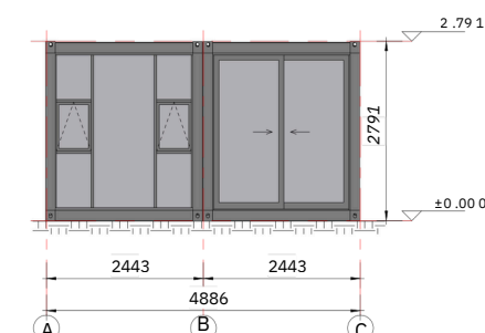
Élévation de la grille 2
