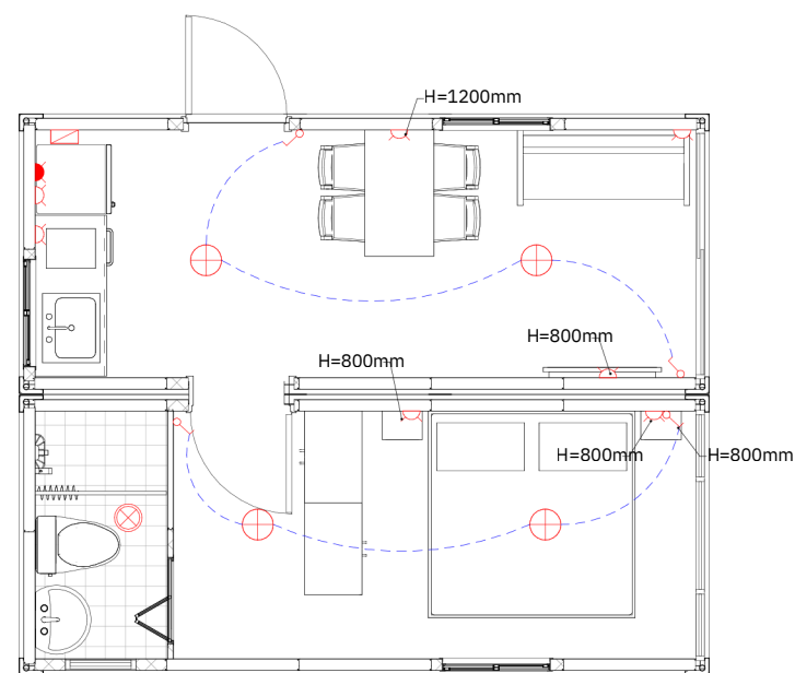
Plan électrique
