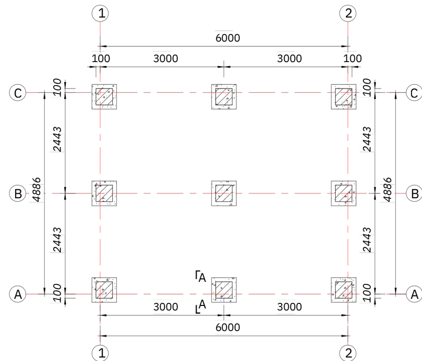
Plan de fondation
