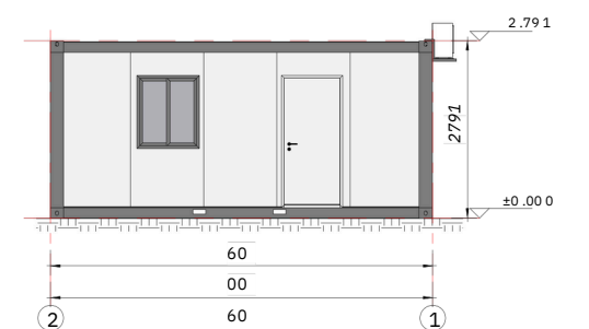
Élévation de la grille C
