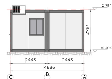
Élévation de la grille 1
