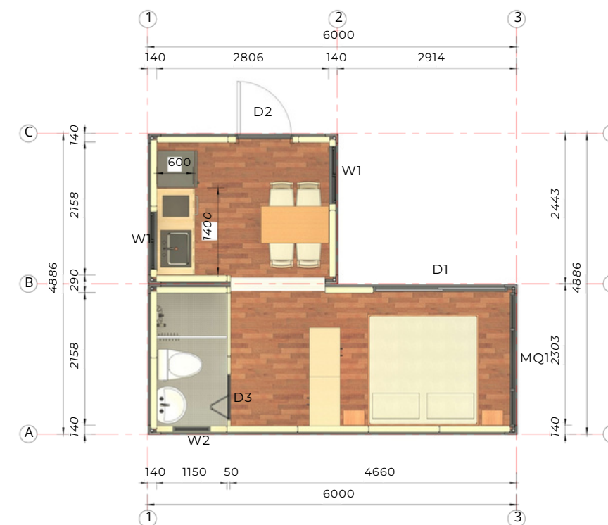
Plan d'aménagement
