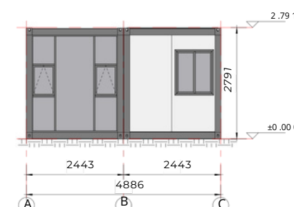
Élévation de la grille 3
