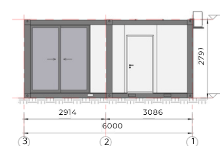
Élévation de la grille C
