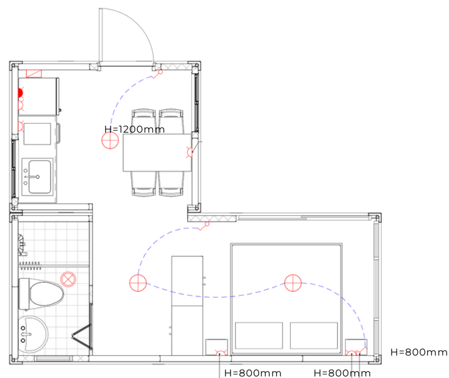
plan électrique
