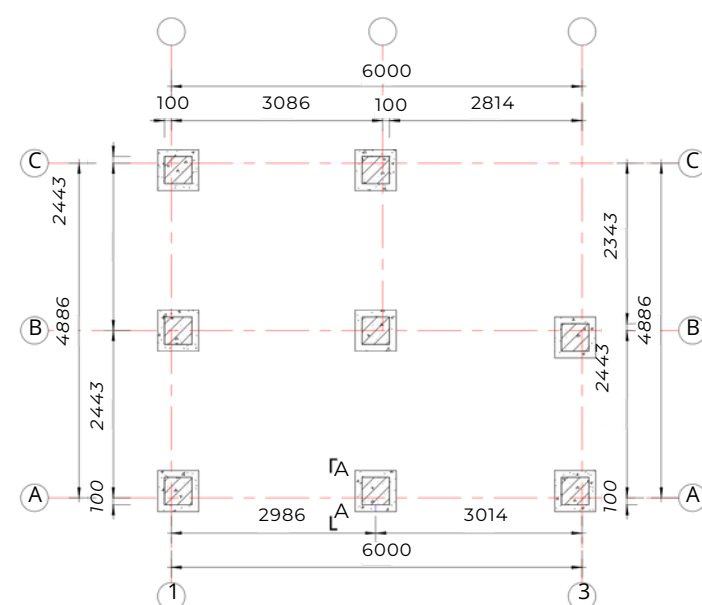
Plan de fondation
